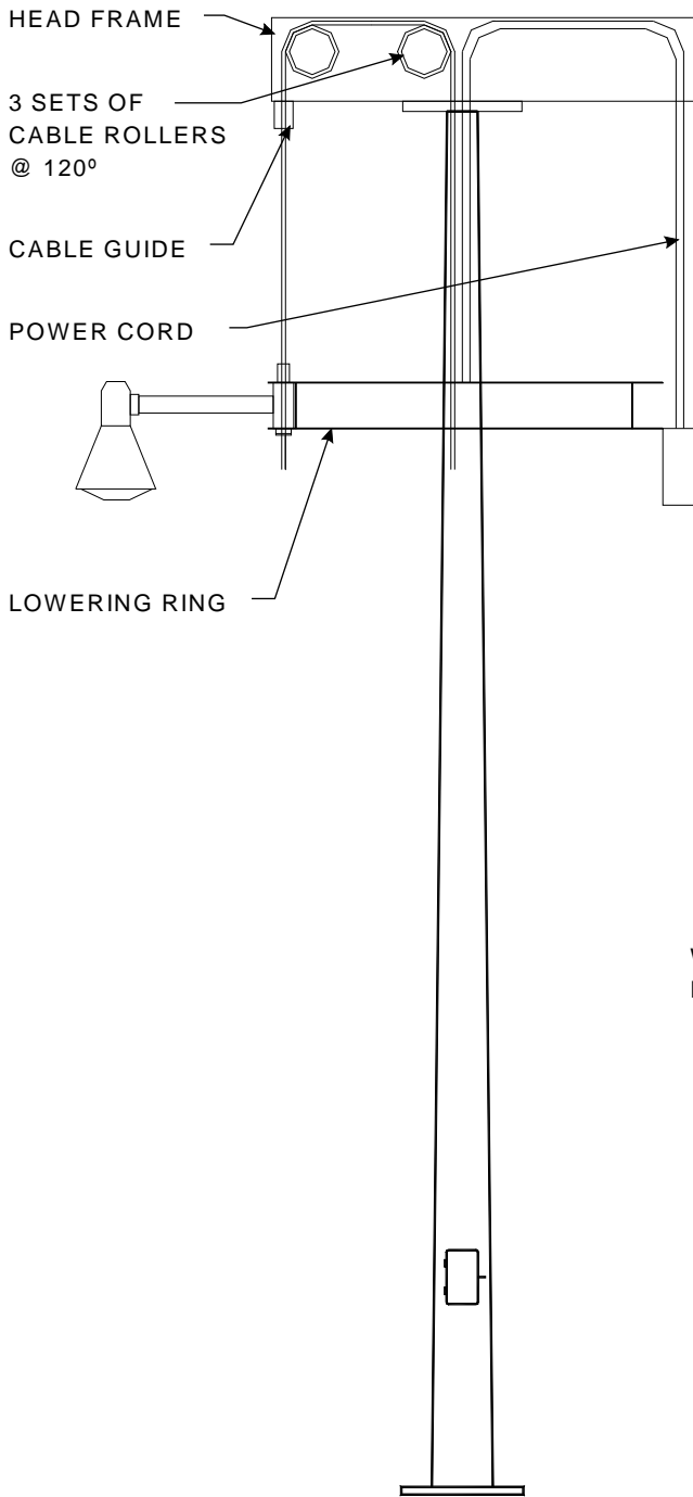
POLE ELEVATION
